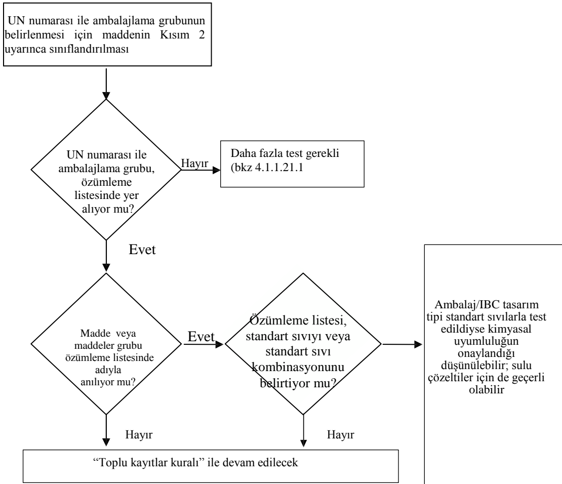
Şekil 4.1.1.21.1: Doldurma maddelerinin standart sıvılara özümlenmesine dair şema
