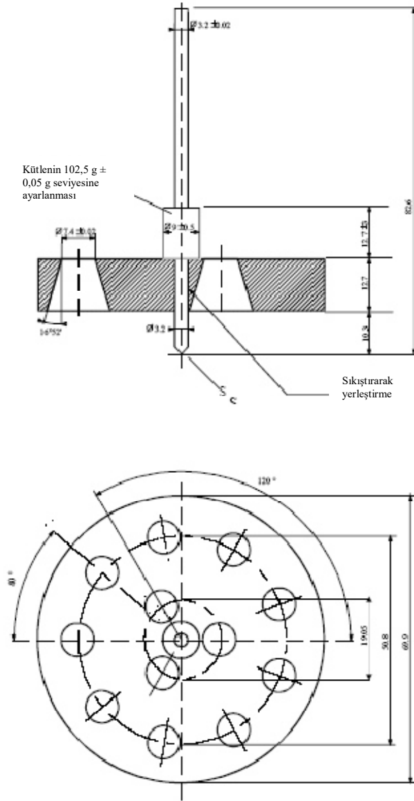
Şekil 1 - Penetrometre
