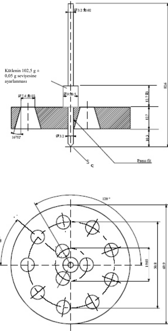
Şekil 1 - Penetrometre
