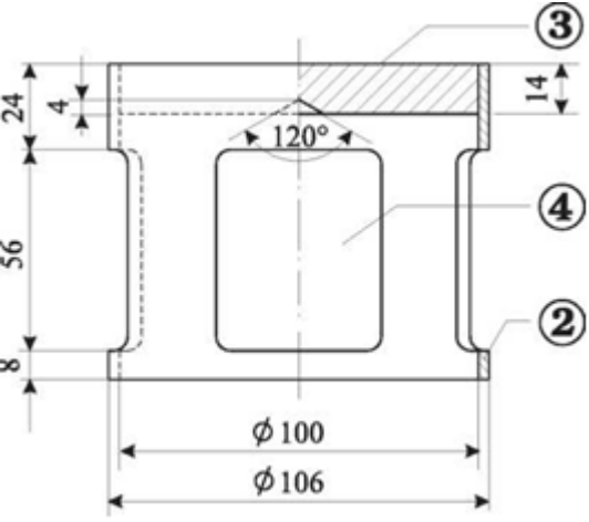
Şekil 1: Çan formunda yük, kütlesi 2220 g, bronz piston üzerinden asılabilen
