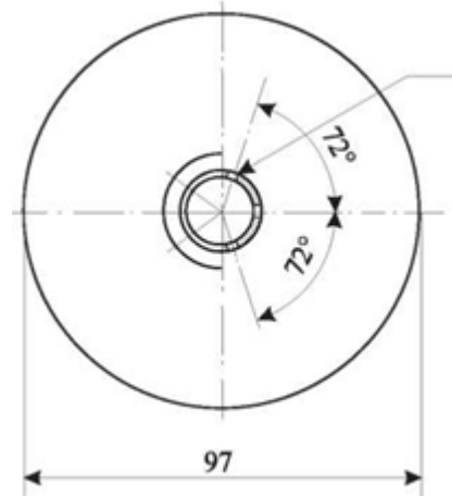
Şekil 3: İçi boş bronz silindir, bir uçtan kapanır, çizim ve kesim boyutları mm olarak
